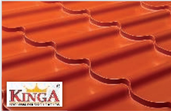
FLORIAN CENTRUM, Blachodachówka Kinga . Ma klasyczny kształt imitujący tradycyjną dachówkę ceramiczną. Długość modułu [mm]: 350. Wysokość tloczenia [mm]: 20.
